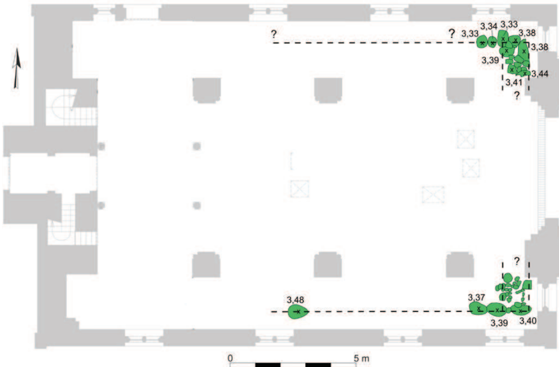
Fig. 5. Plattegrond van het schip van de Catharinakerk met daarin aangegeven de aangetroffen resten van de fundering van veldkeien van een houten kerk. Voor zover valt na te gaan is de bakstenen kerk nauwsluitend om de houten kerk heen gebouwd. De getallen zijn de hoogtewaarden in m +NAP. Tekening P. den Hengst.
